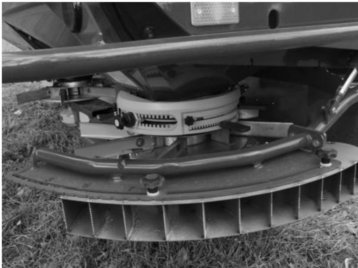
Wielopłytkowy deflektor ExactLine zamontowany na rozsiewaczu Exacta-HL, stosowany do siewu granicznego, (fot. ITP-PIB)
